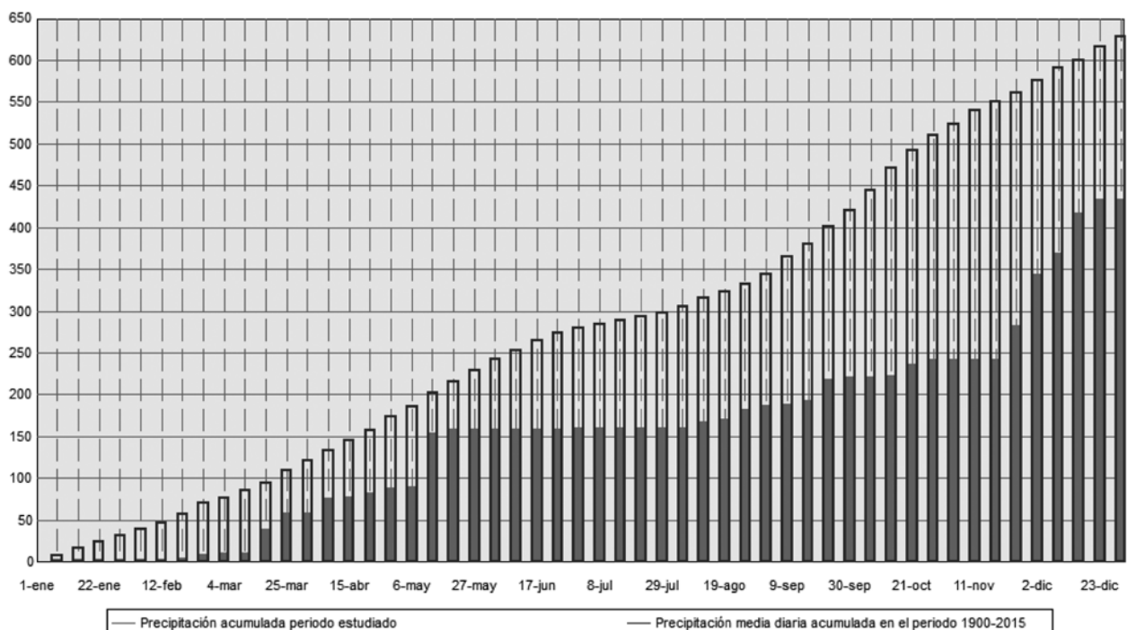
Precipitación acumulada (mm) enero - diciembre 2016 en ATZENETA DEL MAESTRAT
